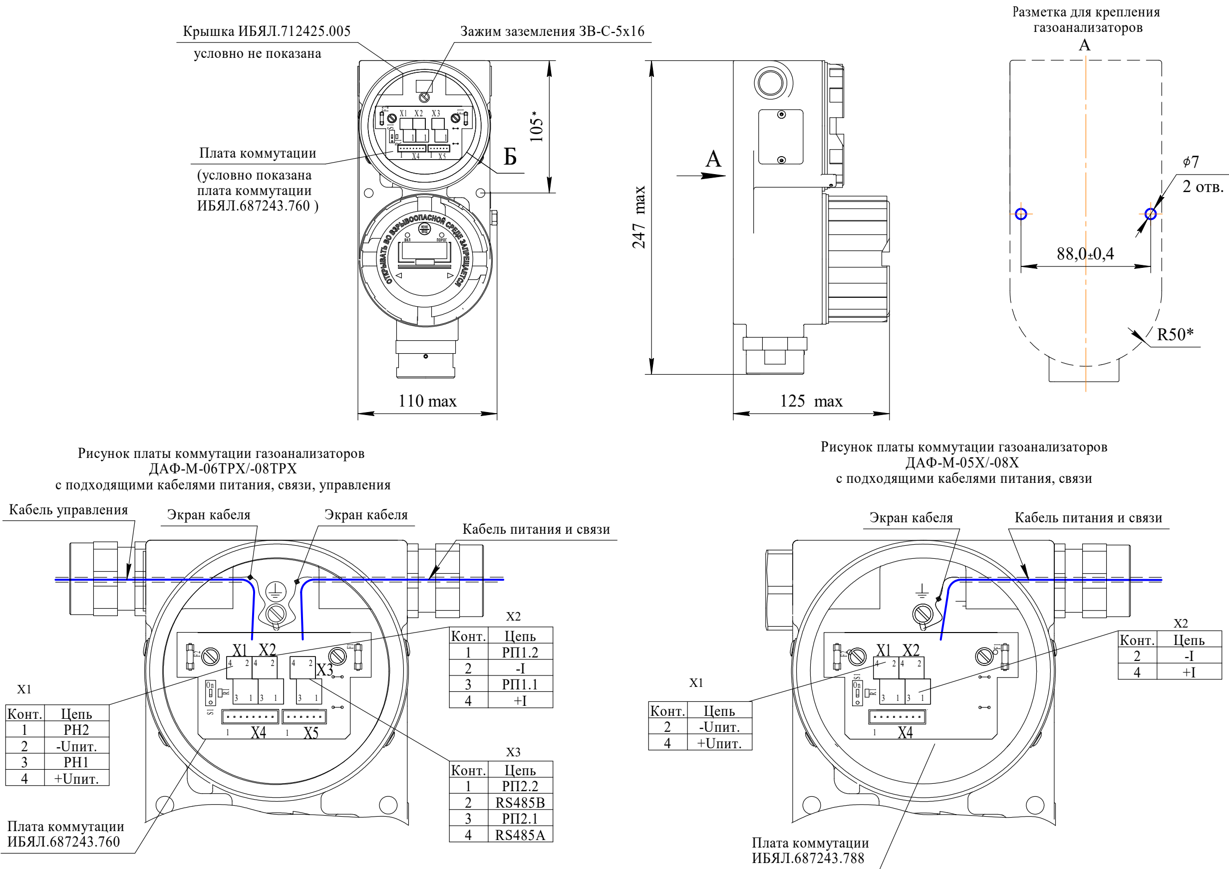
Рисунок К.2 – Монтажный чертеж газоанализаторов ДАФ-М-05Х/-08Х/-06ТРХ/-08ТРХ
