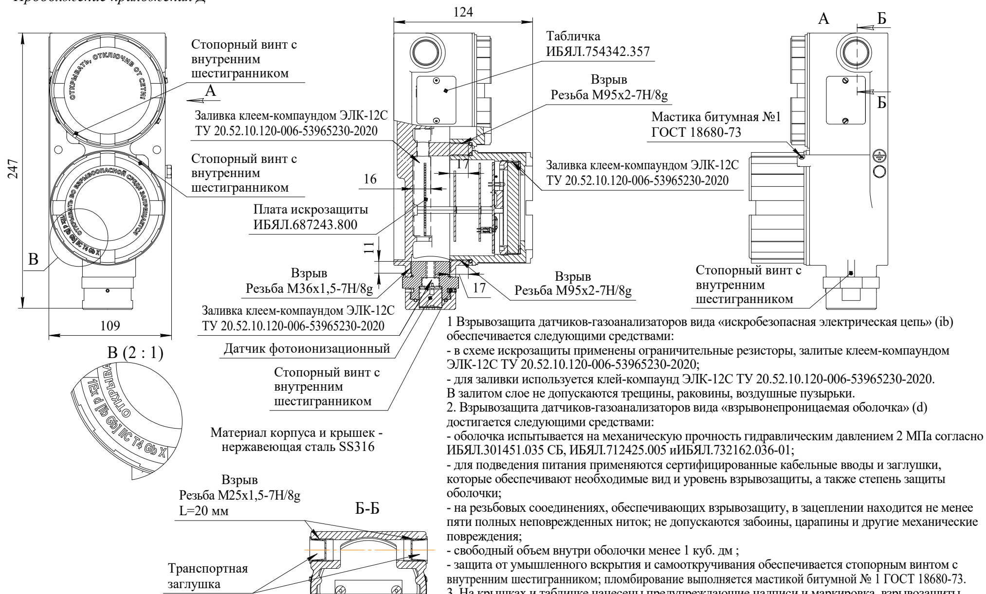
Рисунок Д.3 – Чертеж средств взрывозащиты датчиков-газоанализаторов ИБЯЛ.413445.003-80 (-85)
