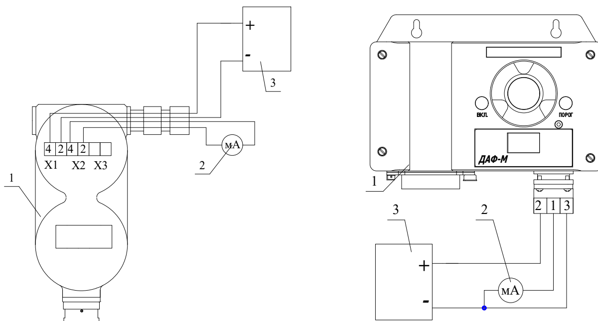
а) ДАФ-М-05Х/-08Х/-06ТРХ/-08ТРХ
