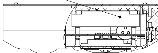
Рисунок Д.1 – Чертеж средств взрывозащиты датчиков-газоанализаторов ИБЯЛ.413445.003
