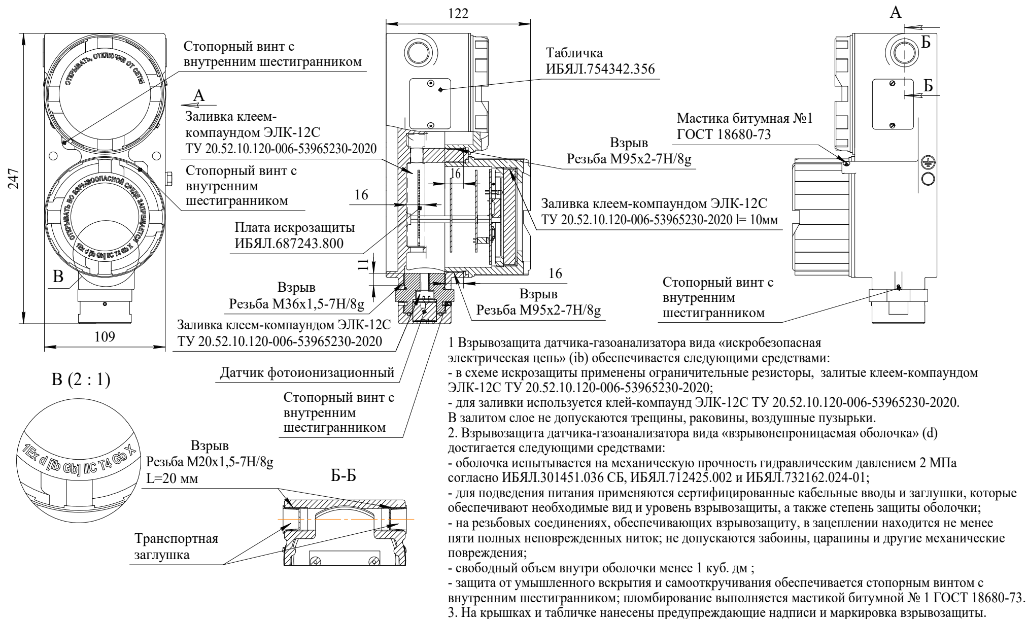
Рисунок Д.2 – Чертеж средств взрывозащиты датчиков-газоанализаторов ИБЯЛ.413445.003-06 (-09)
