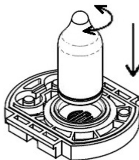
Рисунок 3.6 – Схема установки УФЛ в КИ
