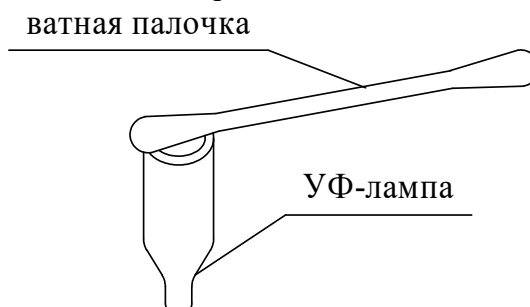
Рисунок 3.5 – Очистка УФЛ
