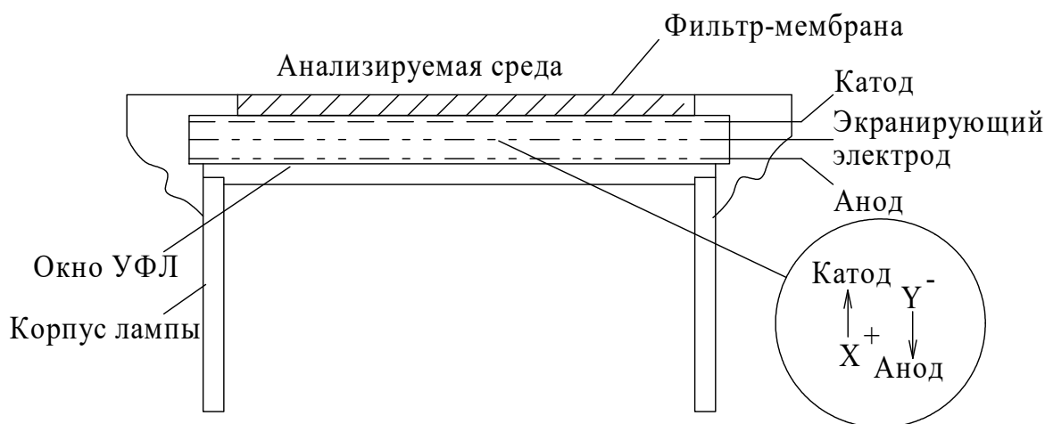
Рисунок 1.2 – Схема работы ФИД
