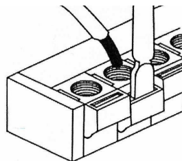
Рисунок 4 – Клеммное соединение
