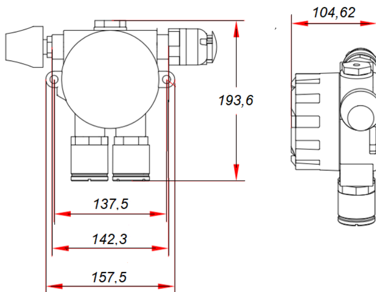
Рисунок 2 – Габаритные размеры прибора
