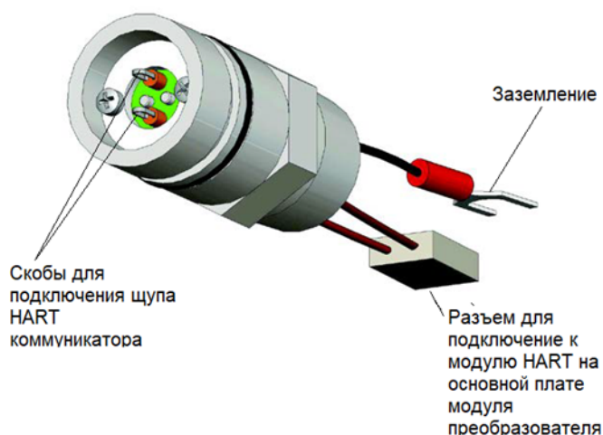
Рисунок 9 – HART-коннектор
