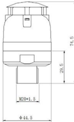
Рисунок 6 – Габаритные размеры маяка
