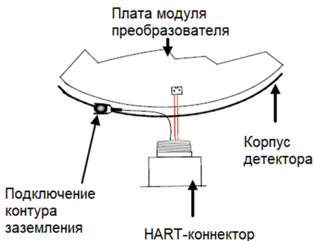
Рисунок 11 – Схема подключения HART-коннектора
