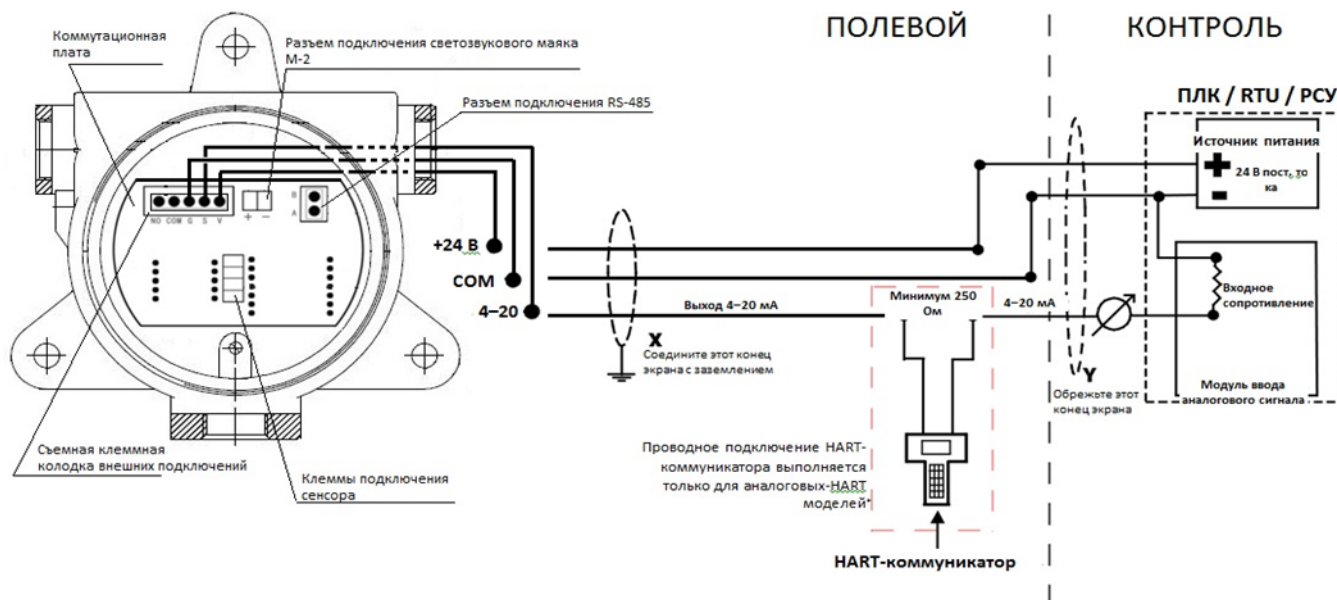
Рисунок 6 – Схема подключения к внешнему источнику питания
