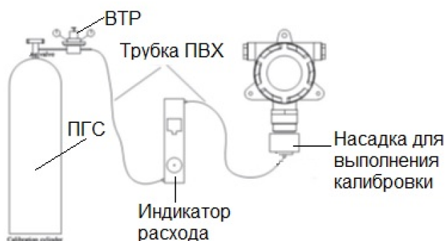
Рисунок 8 – Схема подключения процесса поверки/калибровки
