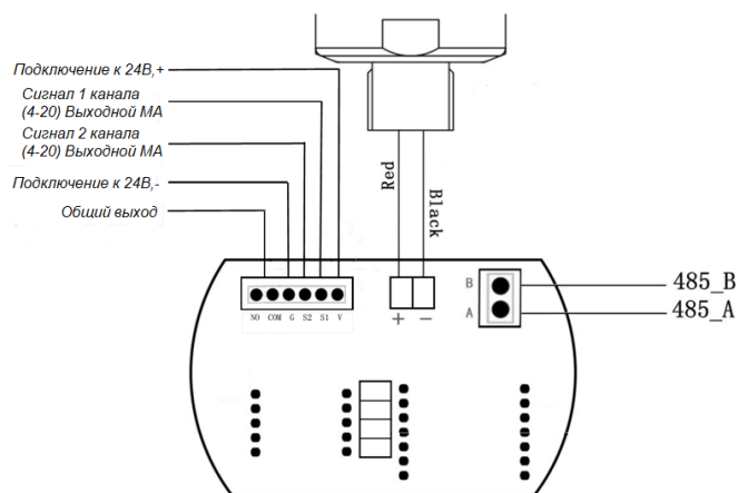
Рисунок 5 – Назначение клемм электрических подключений
