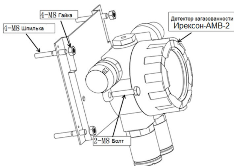
Рисунок 3 – Способ крепления прибора на стене
