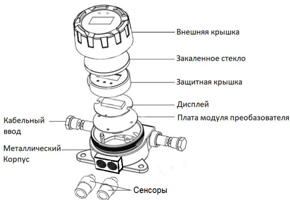
Рисунок1 - Устройство прибора
