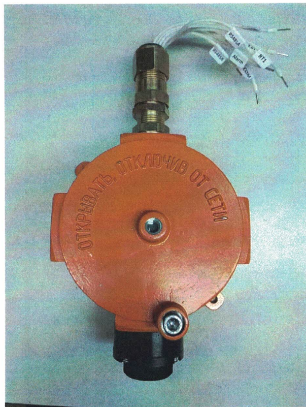
Рисунок 1 - Общий вид газоанализаторов ИГМ-10ИК и ИГМ-10Э
