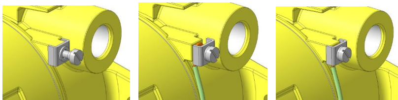
а) ослабить винт б) вставить провод в) затянуть винт Рисунок 20 – Заземление корпуса газоанализатора
