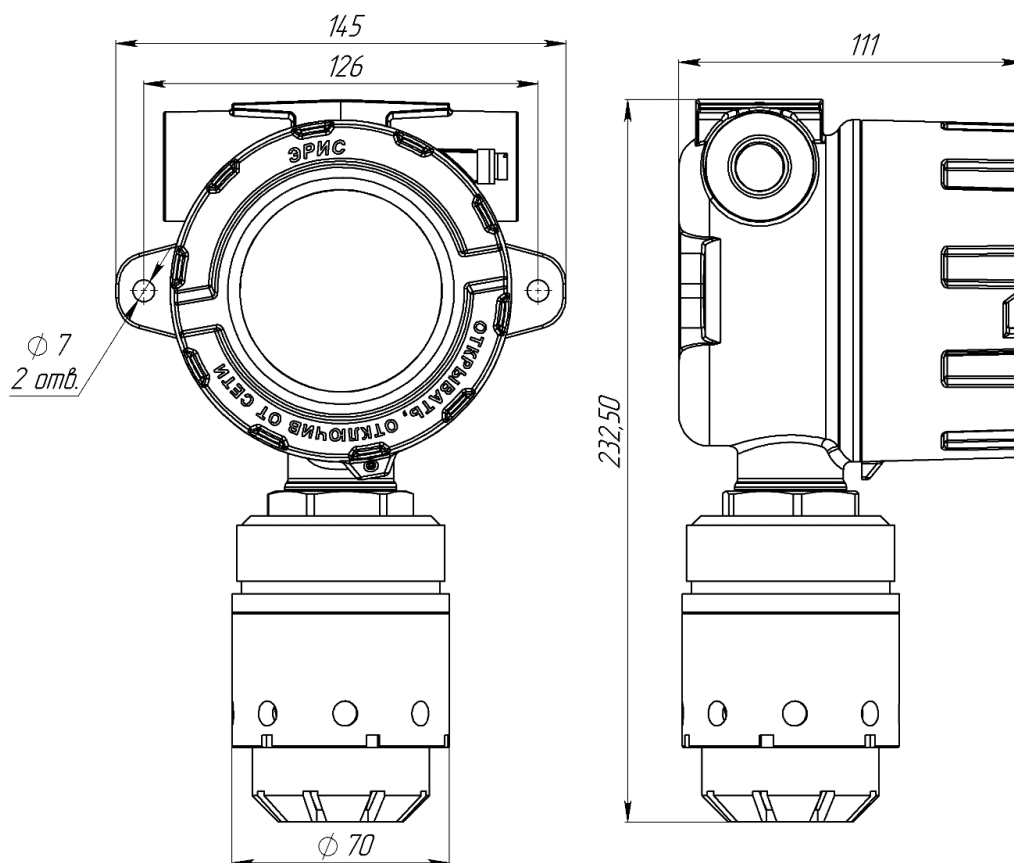
Рисунок 2 – Габаритные размеры Advant 2
