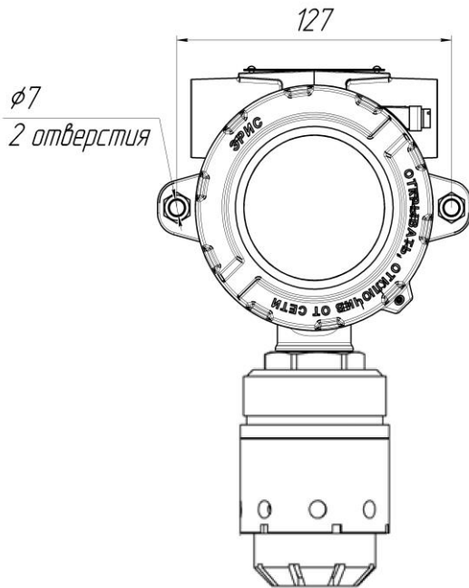
Рисунок 6 – Монтажные размеры
