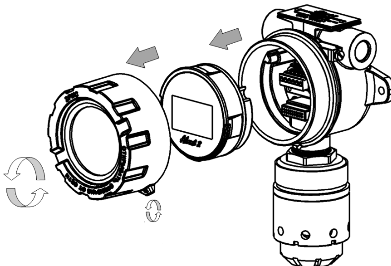
Рисунок 21- Схема разбора газоанализатора
