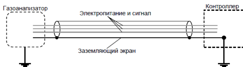
Рисунок 19– Заземление экранированного кабеля
