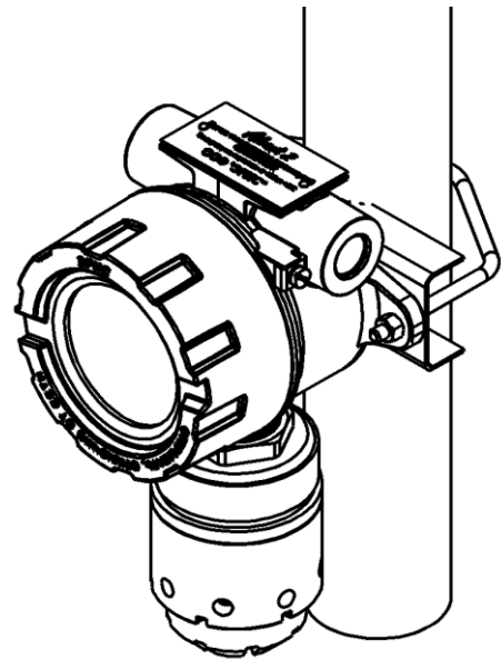
Рисунок 9 – Вид газоанализатора, установленного на трубу
