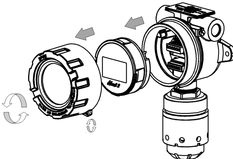
Рисунок 14 – Схема разбора Advant 2
