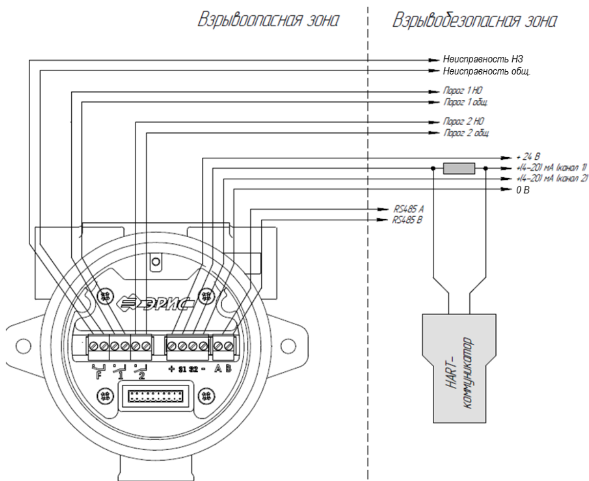
Рисунок 18 – схема подключения газоанализатора Advant 2 с реле и с подключением HART по токовой петле ( R_n = 250 \text{ Ом} )
