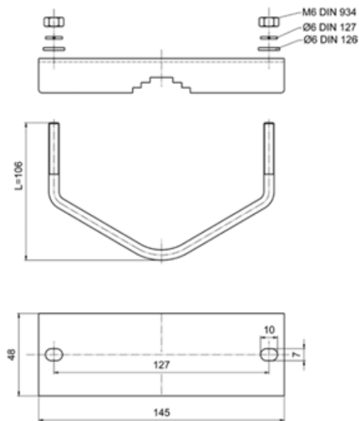
Рисунок 8 – Вид крепления для установки на трубу
