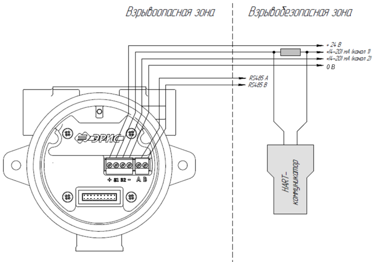
Рисунок 16 –схема подключения газоанализатора Advant 2 с подключением HART по токовой петле ( R_n = 250 \text{ Ом} )
