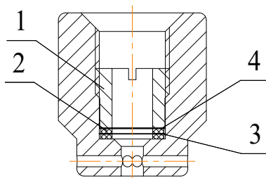
1 – втулка; 2 – прокладка; 3 – шайба; 4 – сетка
