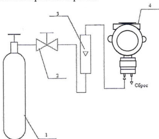
Рисунок 1 - Схема подачи ГС на вход газоанализатора при проведении поверки
