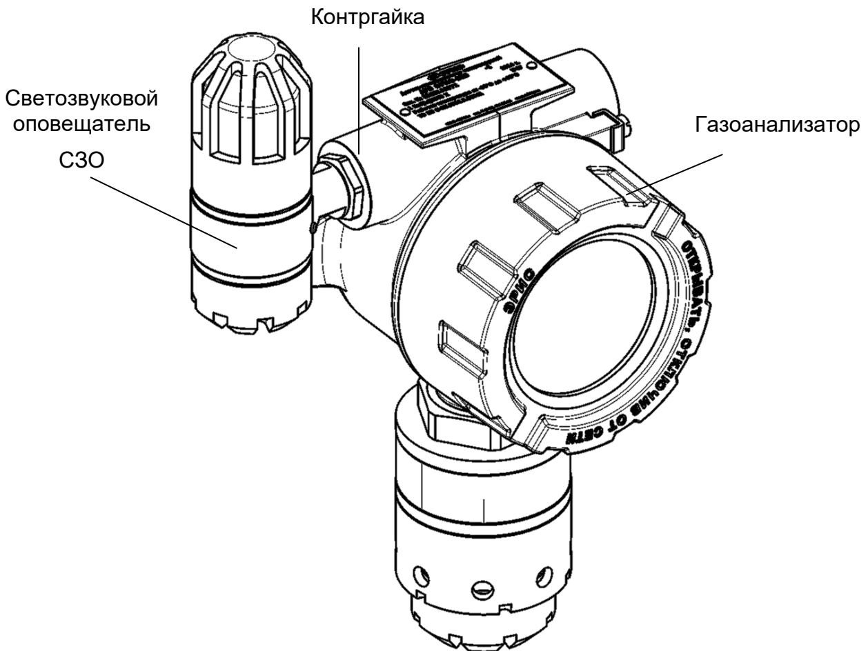
Рисунок 26 – Внешний вид газоанализатора со светозвуковым оповещателем С30
