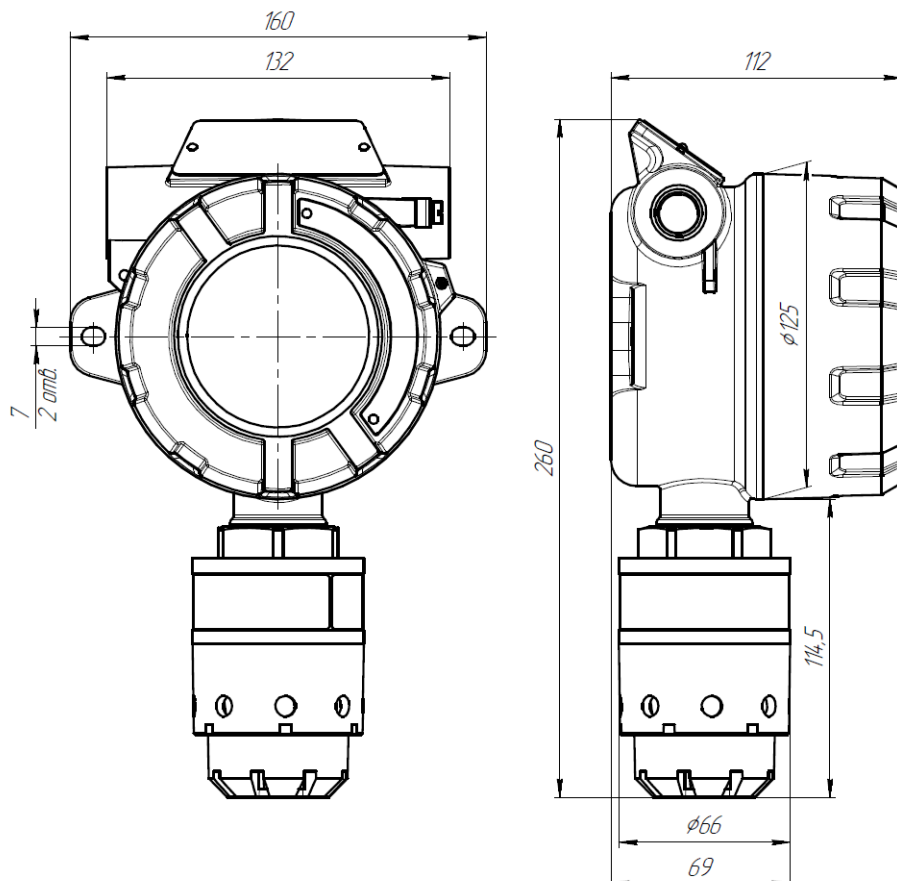
Рисунок 3 – Габаритные размеры ДГС ЭРИС-230 в корпусе типа А
