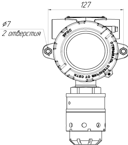
Рисунок 8 – Монтажные размеры
