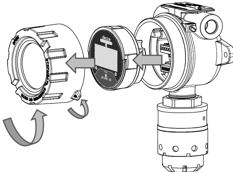
Рисунок 16 – Схема разбора ДГС ЭРИС-230
