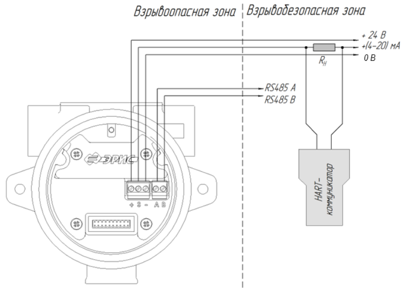
Рисунок 17 – 3-проводная схема подключения газоанализатора ДГС ЭРИС-230 без реле с подключением HART по токовой петле ( R_H = 250 \text{ Ом} )
