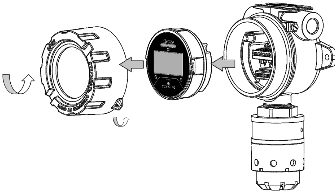
Рисунок 23- Схема разбора газоанализатора
