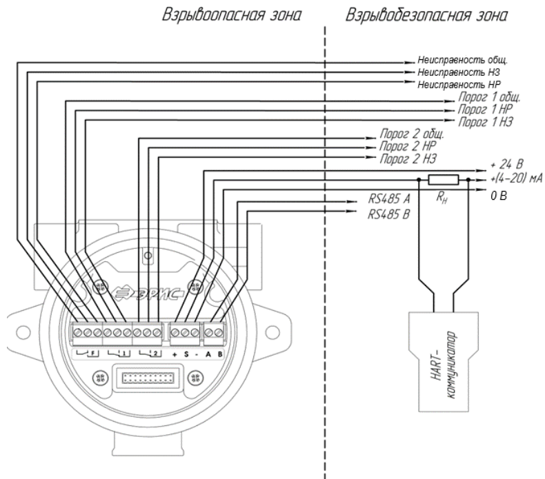
Рисунок 18 – 3-проводная схема подключения газоанализатора ДГС ЭРИС-230 с реле с подключением HART по токовой петле. НР - нормально разомкнутый контакт; НЗ - нормально замкнутый контакт. ( R_H = 250 \text{ Ом} )
