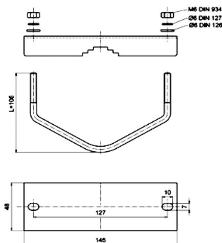
Рисунок 10 – Вид крепления для установки на трубу
