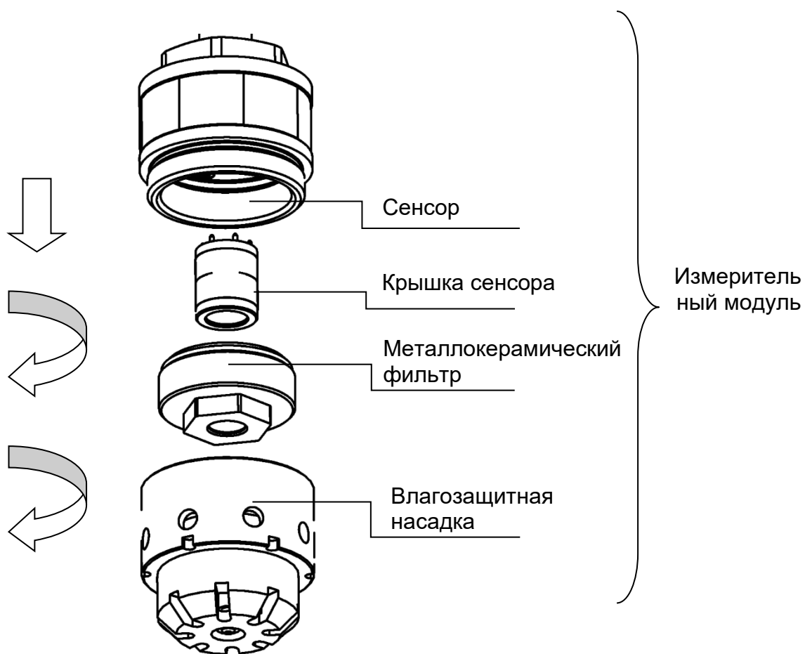
Рисунок 25 – Схема разборки измерительного модуля
