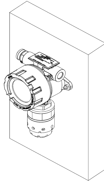
Рисунок 9 – Вид газоанализатора, установленного на стену
