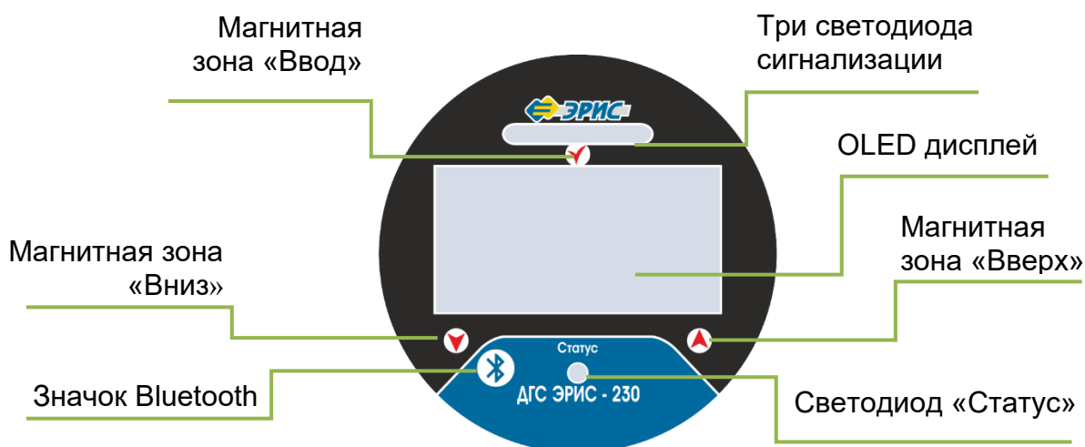
Рисунок 6 – Лицевая панель ДГС ЭРИС-230
