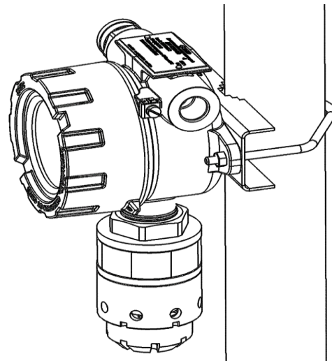
Рисунок 11 – Вид газоанализатора, установленного на трубу
