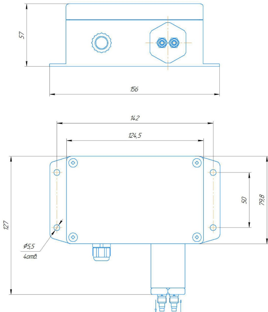
Рисунок 1. Габаритный чертёж прибора
