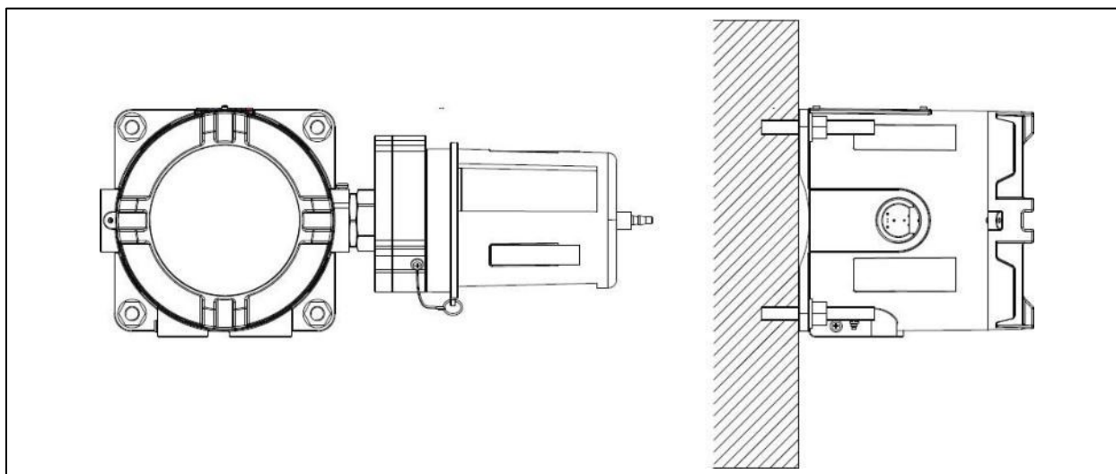
Рис 6: Монтажный чертеж на плоскости
