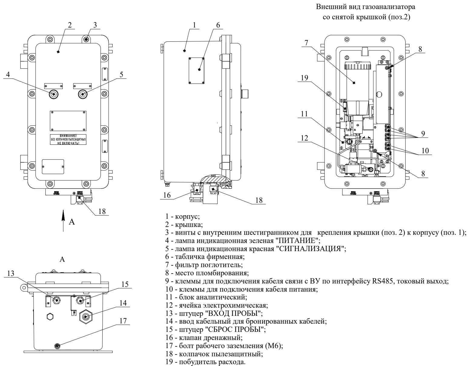
Рисунок 1.1 - Датчики-газоанализаторы паров КРТ ДАРТ ИБЯЛ.413411.054-04. Внешний вид
