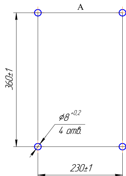
Разметка для крепления газоанализатора
